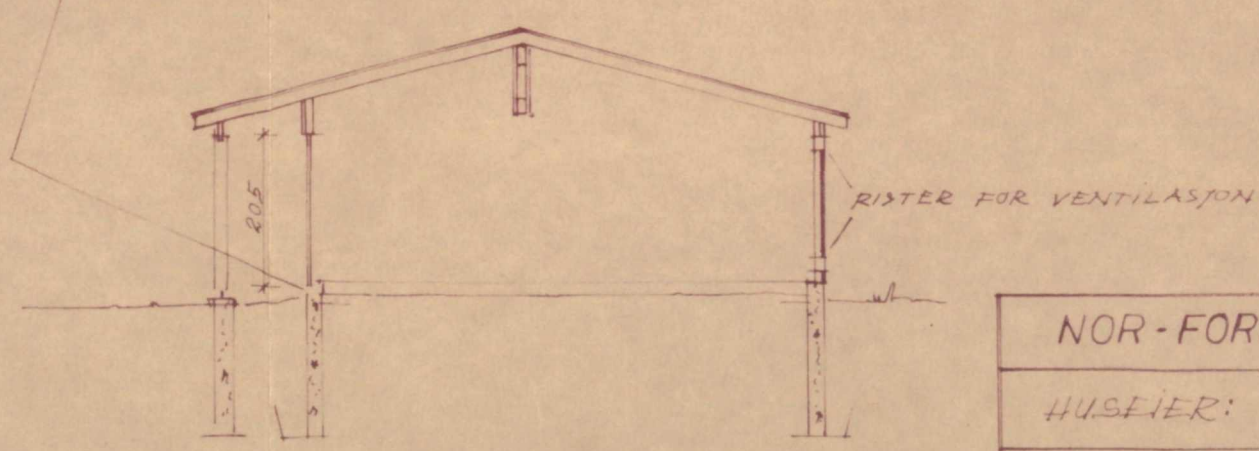
SNITT
